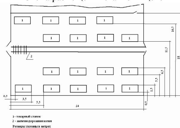
Схема размещения станков в цехе
